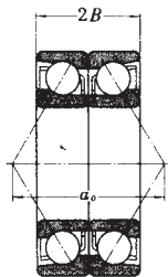
背面組合 (DB)
