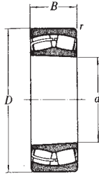
錐形內孔
